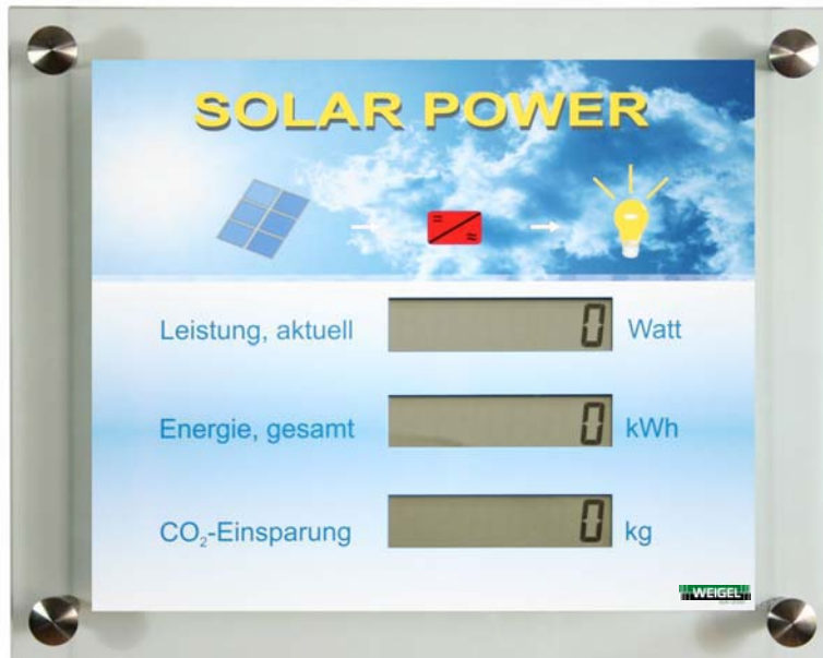
WGA-500si Standardlayout „Himmel mit PV-Symbolik“
