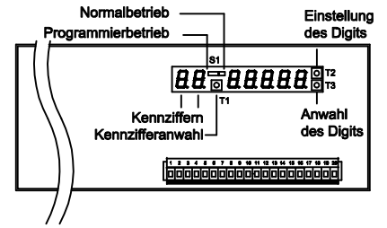
Rückansicht
